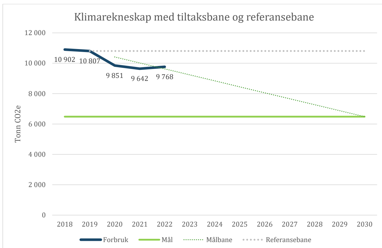
Figur 3: Helse Førde sitt CO 2 e-utslepp med tiltaksbane og referansebane.
